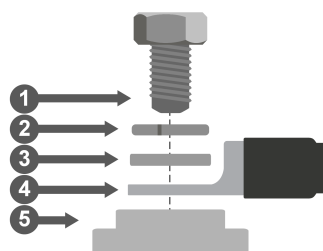
Anschluss der Batteriekabel
