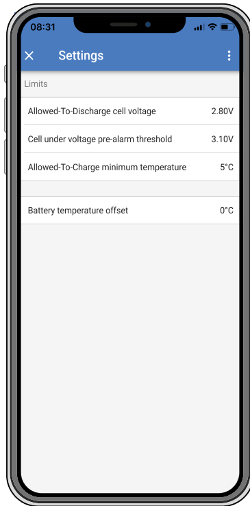
VictronConnect-Batterieeinstellungen
