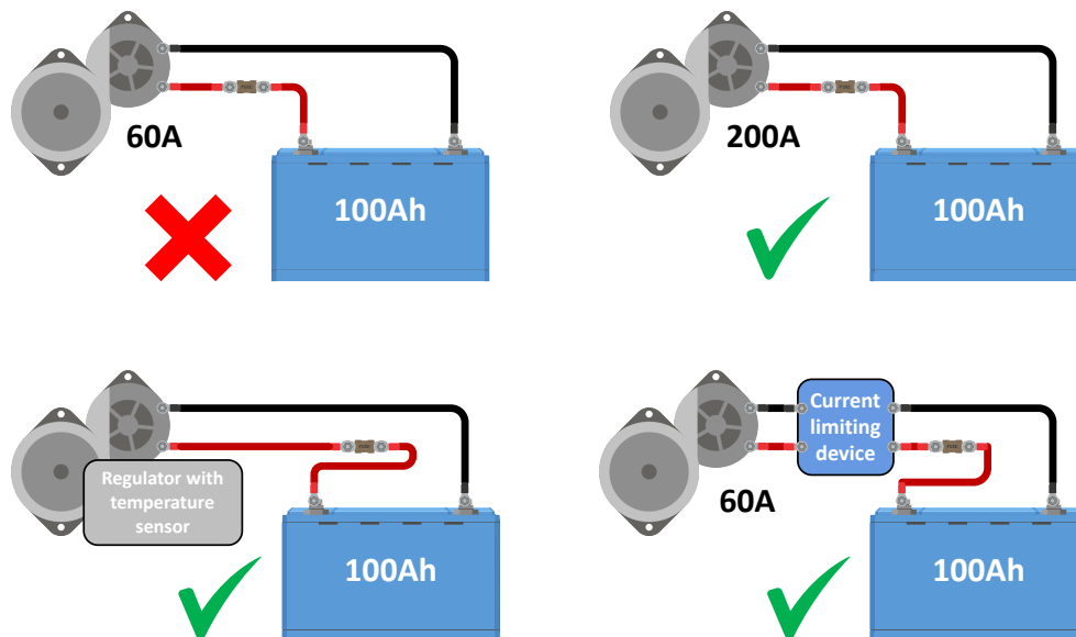
Aufladen der Lichtmaschine
