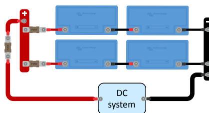
Mehrere Batterien in Reihe/parallel
