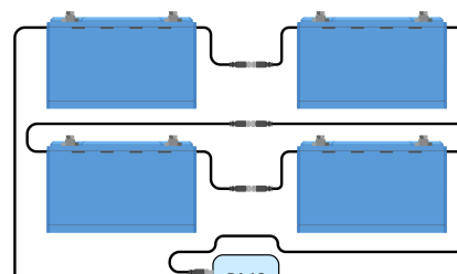
BMS-Anschluss für mehrere Batterien
