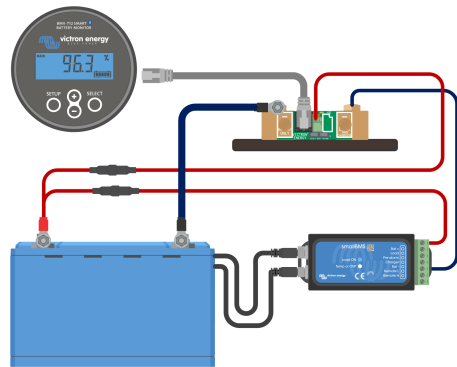
Das Stromkabel des Batteriemonitors ist mit dem BMS verbunden
