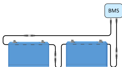
BMS-Anschluss für zwei Batterien (mit optionalen Verlängerungskabeln)
