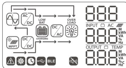
Abb. 22: LCD- Anzeige-Symbole
