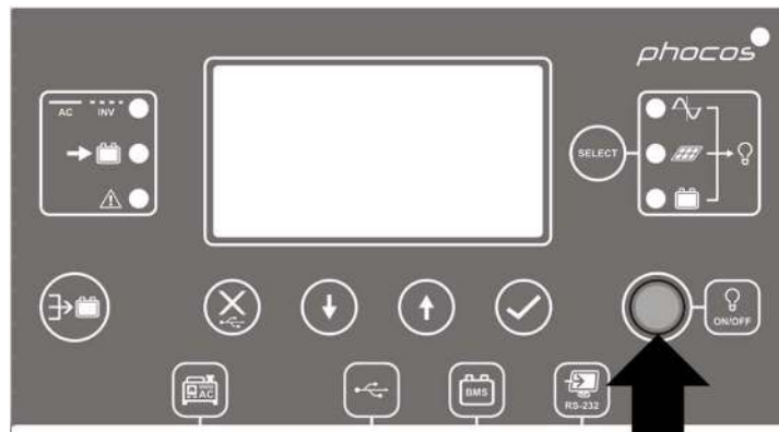
Abb. 20: Anzeigeeinheit Ein-/Ausmacher Position für AC-Ausgang
