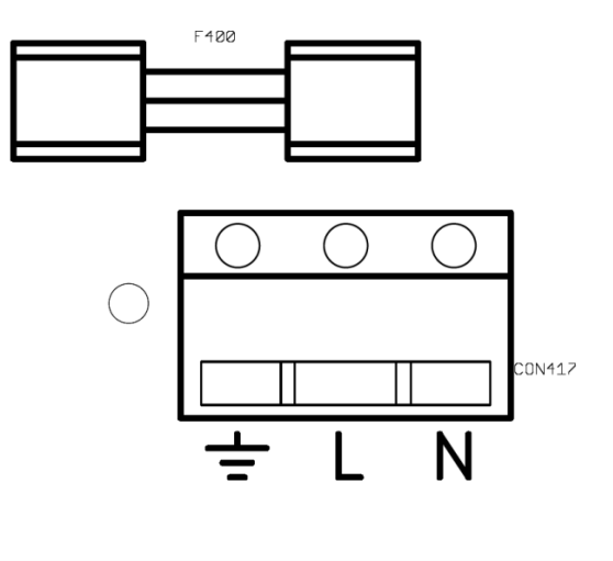
Abbildung 2 Netzeingangsklemme
