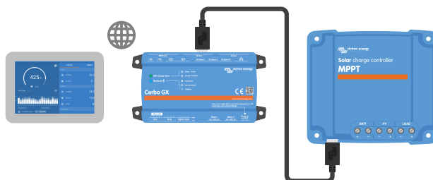
Verbindung der VictronConnect App über LAN oder das Internet (VRM Portal) mit einem GX-Gerät (z. B. einem Cerbo GX)
