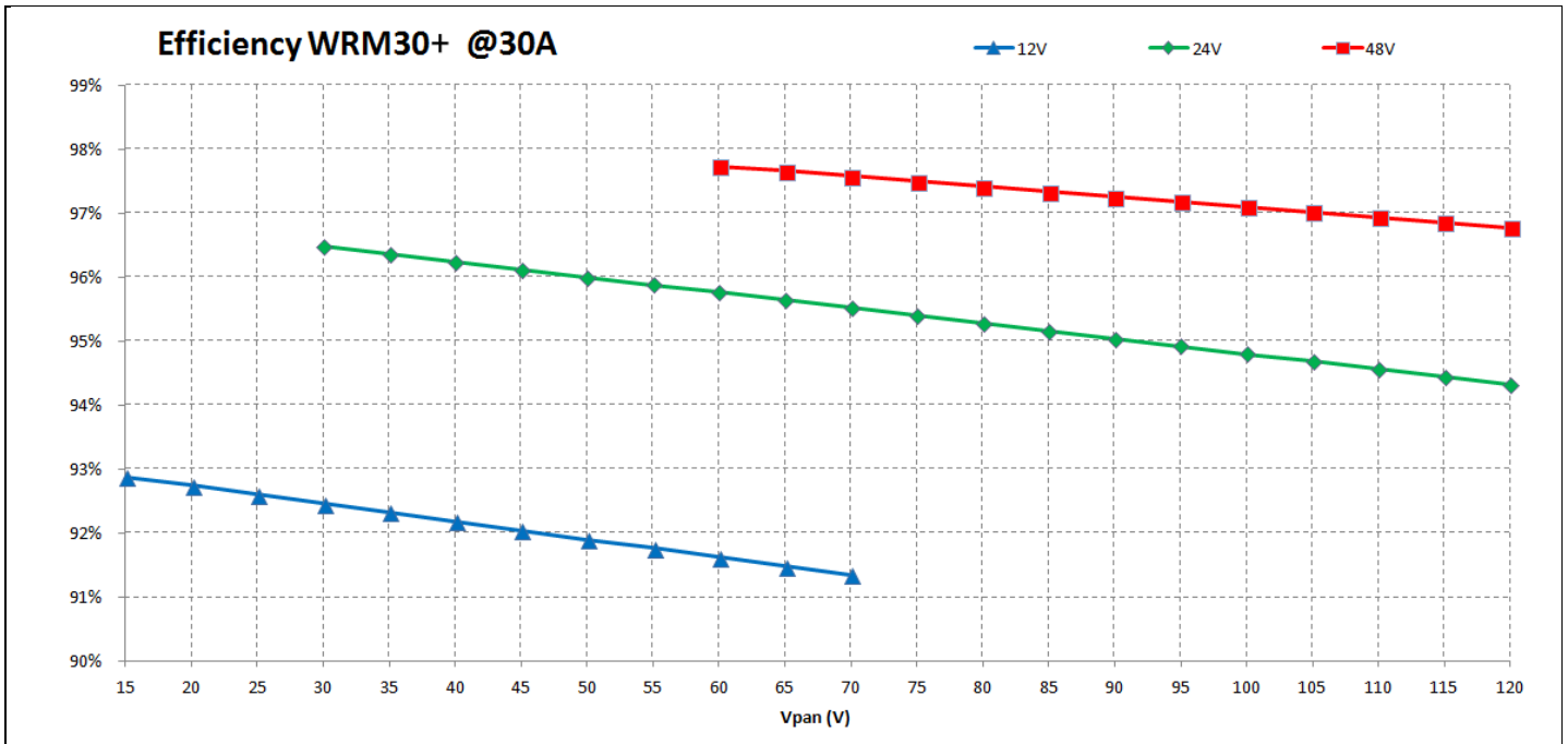
Graf. 2 Effizienz
