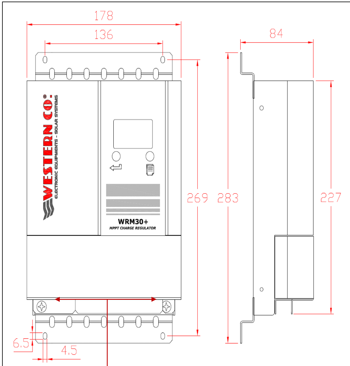
Fig. 4 Dimensions (mm)
