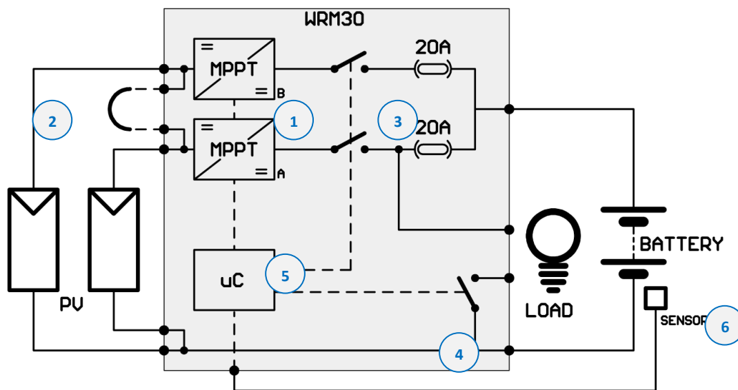
Abb. 1 Prinzipschema
