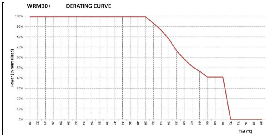
Graf. 3 Derating-Kurve
