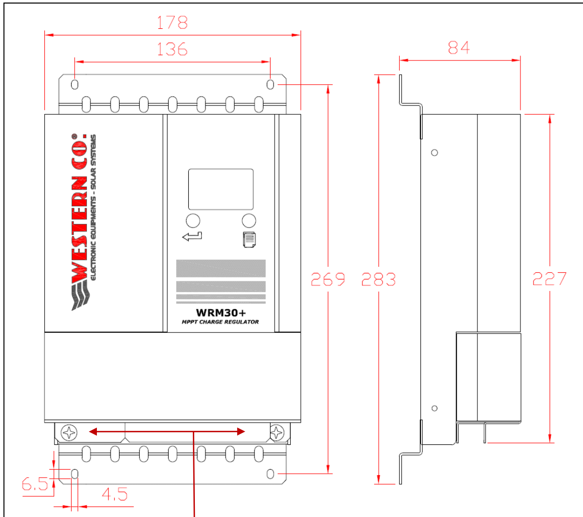
Fig. 4 Dimensioni (mm)
