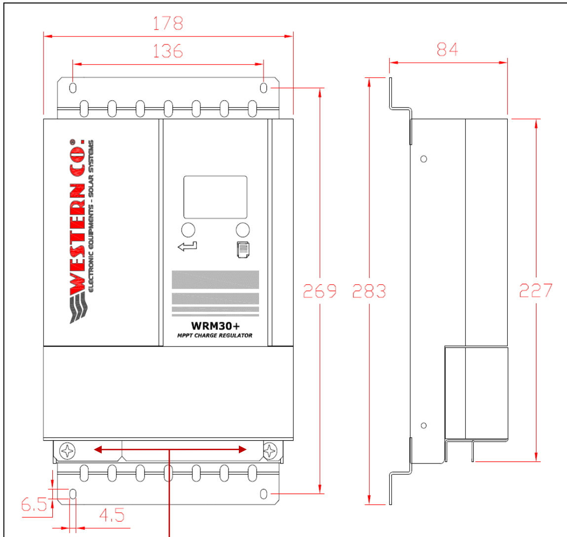
Abb. 4 Ausmaße (mm)
