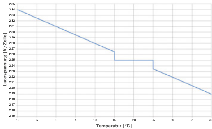
Abb. 6-1: Temperaturabhängige Anpassung der Ladeerhaltungsspannung
