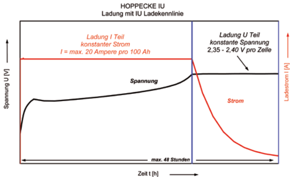
Abb. 9-1: Kennlinie IU
