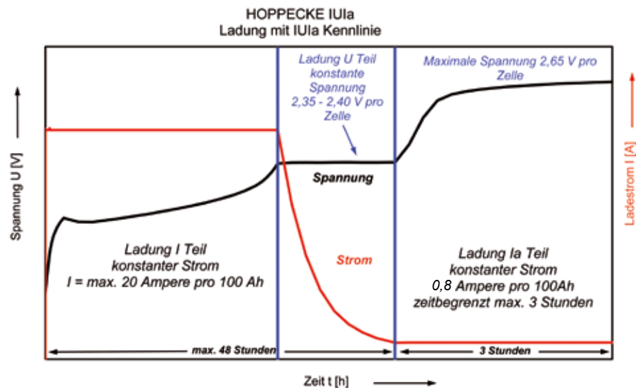
Abb. 9-2: Kennlinie IUa
