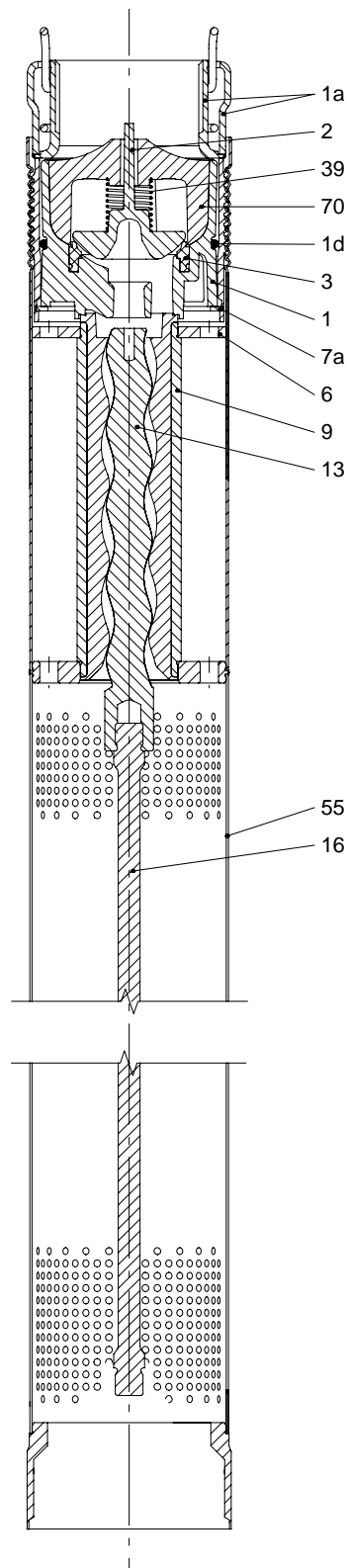
Fig. 26 Example: SQF 1.2-2
